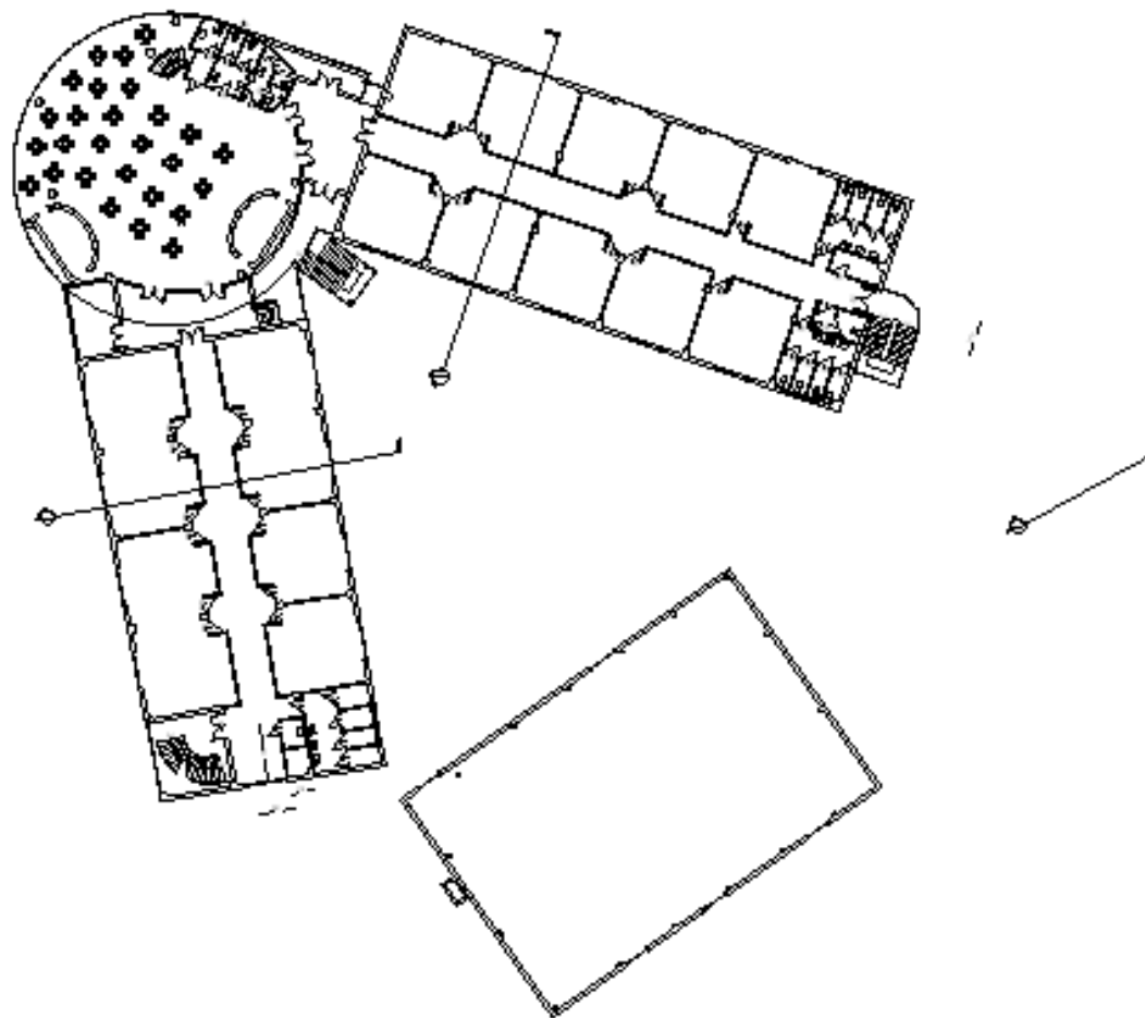
Pianta Piano Secondo – Sala ristorante / Aule didattiche
